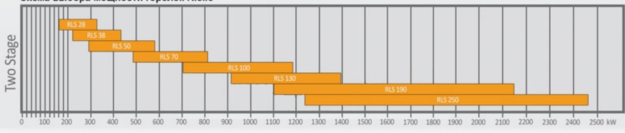
Схема выбора мощности горелок Riello
